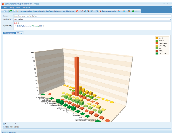
Wykres typu manhattan
